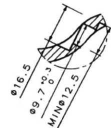
Detail C Scale: 1:1
