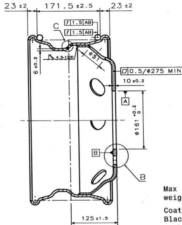
Section view A-A Scale: 1:4
